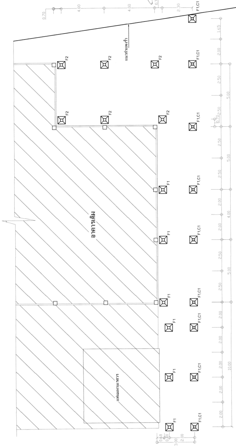
แปลนฐานราก | มาตรฐาน 1 : 100
